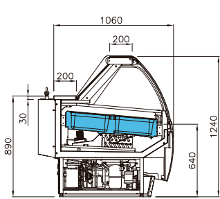
PARGL 3L1 gelados ice cream crème glacée helados
