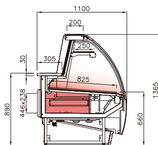
PAAVH aquecida ventilada c/ humidade ventilated dry heated w/ humidity chaude ventilée avec humidité caliente ventilada con humedad
