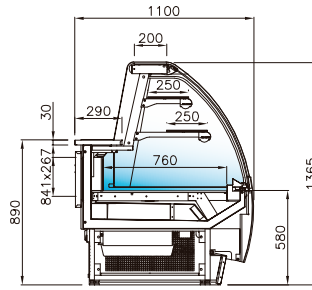
PARPGV 3M2 ventilada com gavetão fan assisted w/ slide-out drawer ventilée avec tiroir ventilada con cajon
