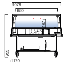
EXPF RV 3M2 ventilada fan assisted ventilée ventilada
